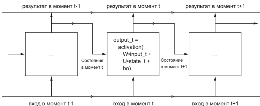
Рис. 6.13. Начальная точка слоя LSTM: слой SimpleRNN
