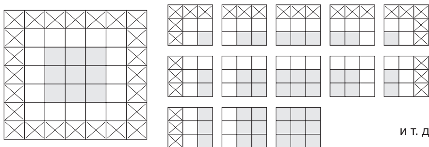
Рис. 5.6. Дополнение входной карты признаков 5 \times 5 , чтобы получить 25 шаблонов 3 \times 3
