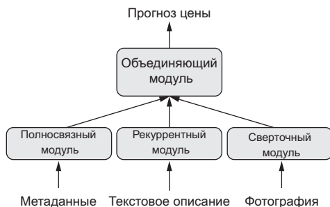
Рис. 7.2. Модель с несколькими входами
