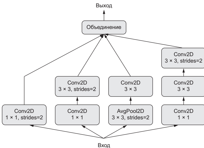
Рис. 7.8. Модуль Inception
